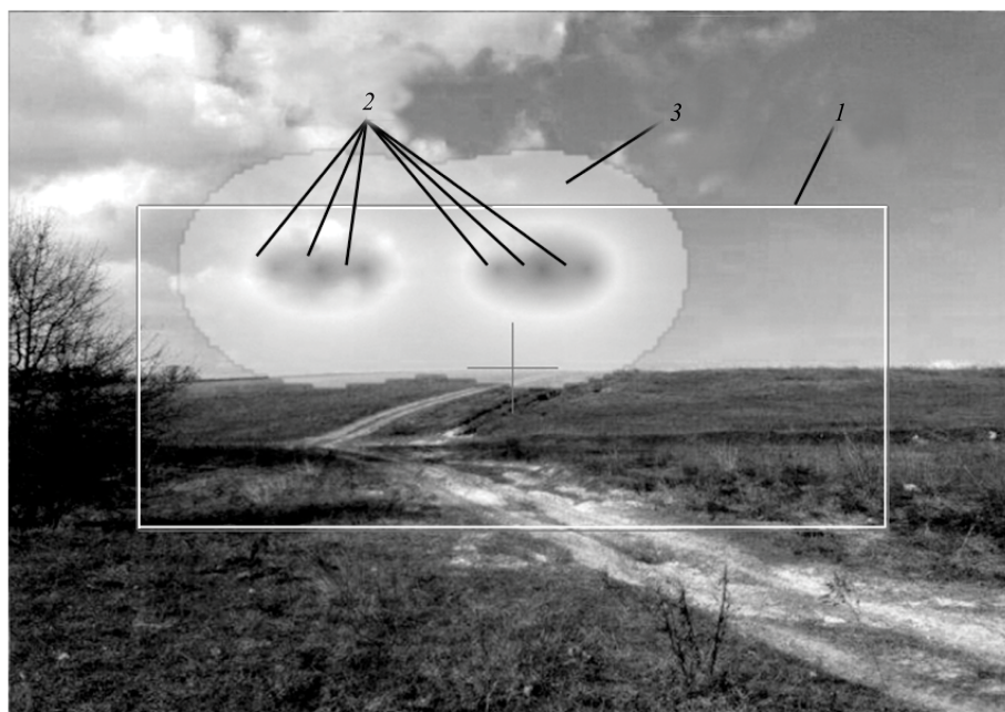
Рис. 2. Визуализация обнаружения облака паров вещества с помощью панорамного ИК ФСТ (облако отображается поверх видеоряда местности):
