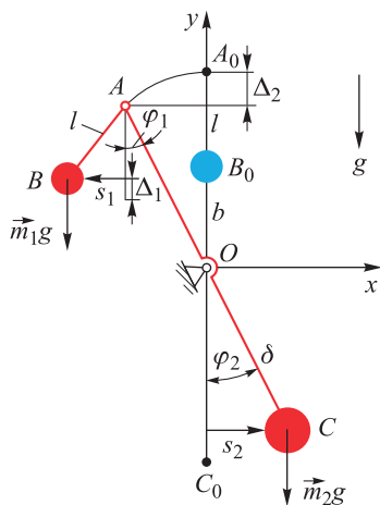
Рис. 5. Механическая модель
