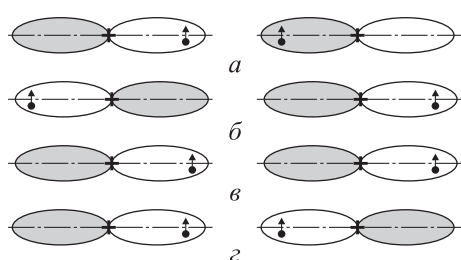
Рис. 3. Схемы, иллюстрирующие случаи, в которых образование связи не происходит
